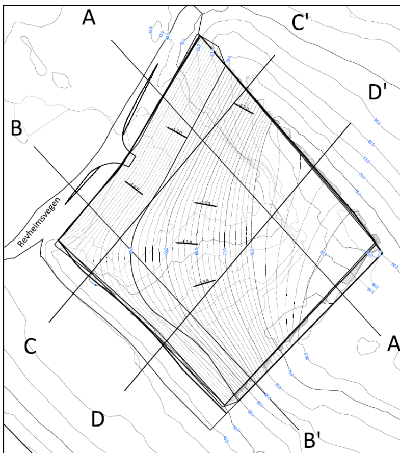
Figur 7-4: Oversikt snitt-teikningar.
