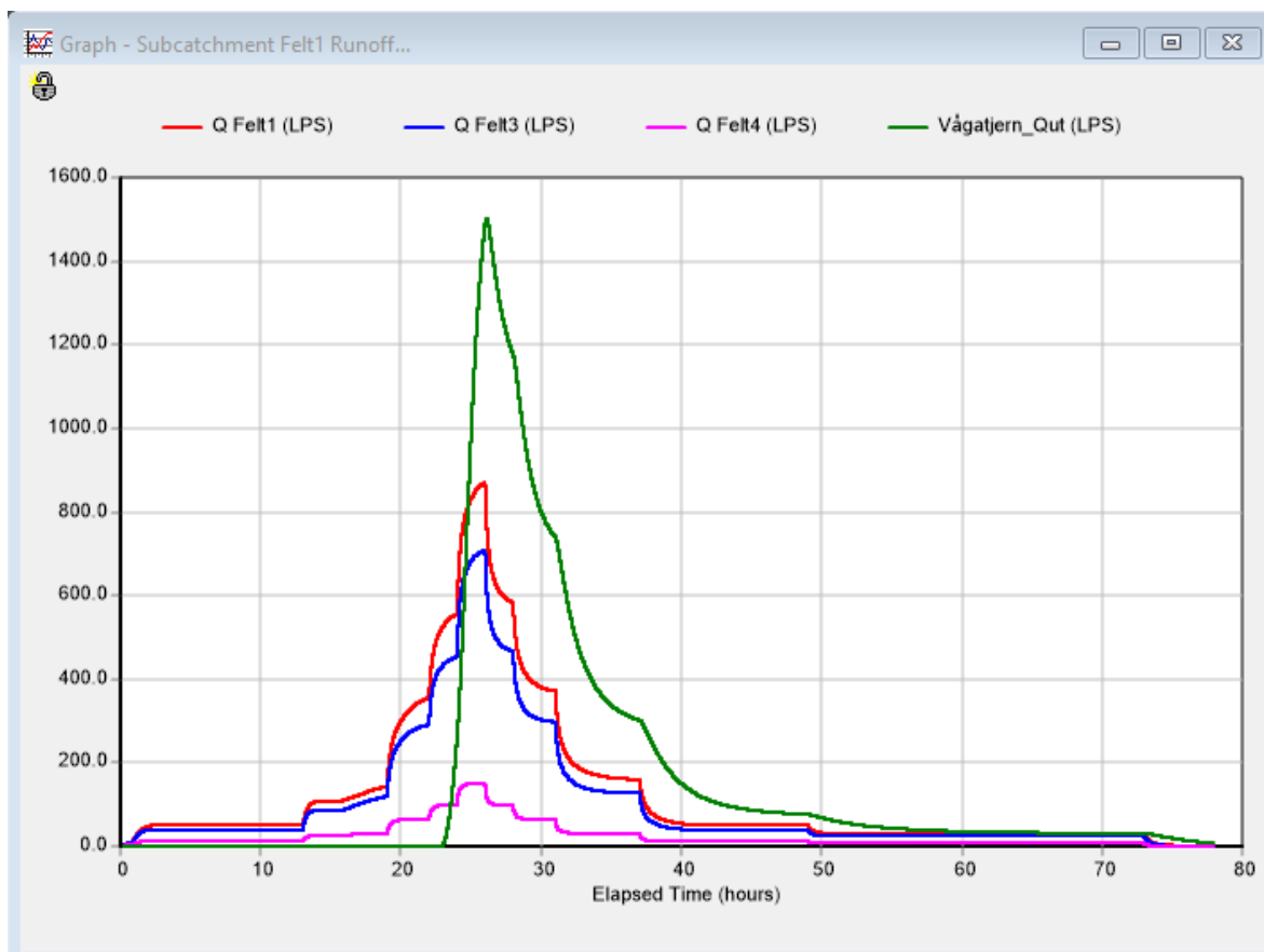
Figur 7: Tilrenning og avrenning til/frå Vågatjøerna for nedbør med 200 års-gjentaksintervall. Grøn kurve er avløp fra Vågatjøerna. Dei øvrige kurvene er tilrenning frå ulike delfelt. Resultat frå modellering i SWMM
