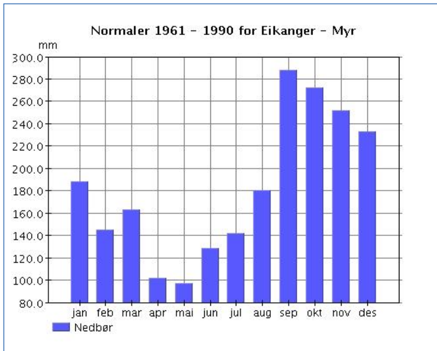
Figur 5. Nedbørsnormal for værstasjonen Eikanger - Myr.
