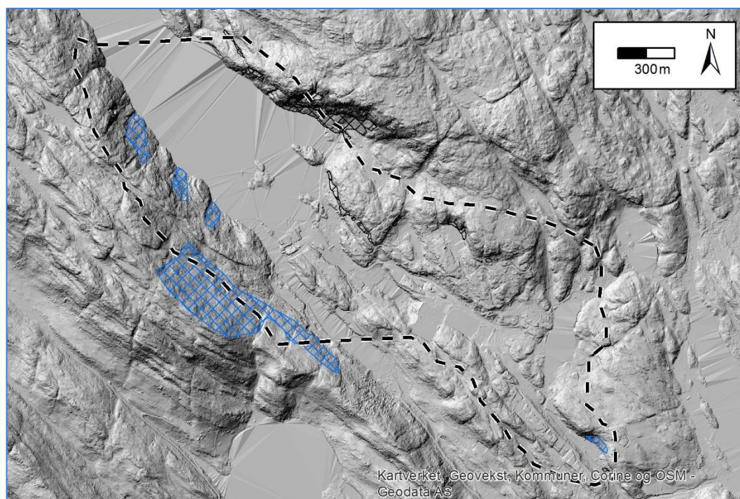
Figur 11. Potensiell løsnemråder for snøskred (blå skravur). Pga. skog i løsenområdene vurderes nominell årlig sannsynligheten for snøskred å være mindre enn 1/5000.
